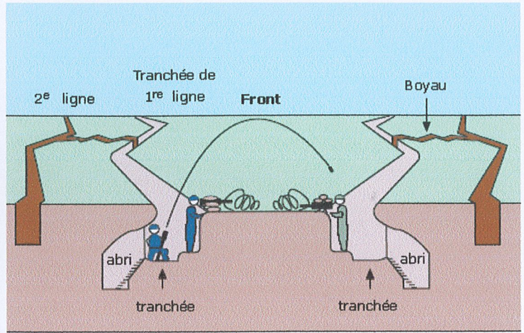
Coupe d'une tranchée
